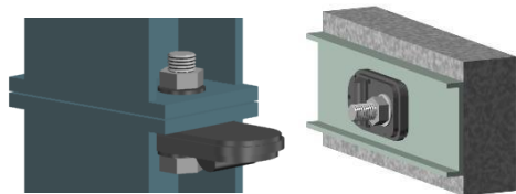
締結ボルト
