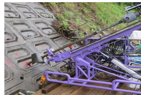
ホーク・ネイリング工法
