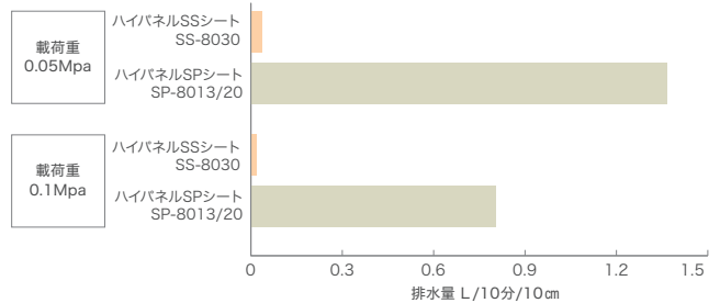
SSシートとSPシートの排水能力比較 (試験方法: ISO12958準拠)
