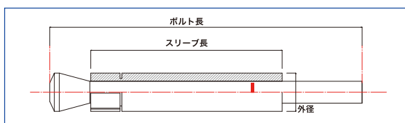
ホーク・カクティアンカー標準図
