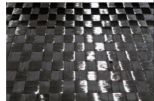
CR200 (2方向高強度炭素繊維) 補修用炭素繊維シート
