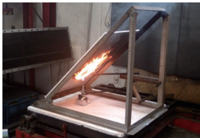
延焼性・自己消火試験
